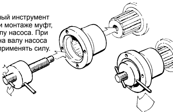
Рис. 7. Монтажный инструмент.
