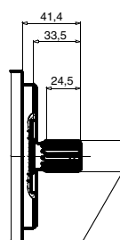
Код вала 3 ШЛИЦЕВОЙ ВАЛ SAE В КЛАСС 1 - J498 b 16/32 d.p. - 13 ЗУБЬЕВ УГОЛ ЗАЦЕПЛЕНИЯ 30° ПЛОСКОЕ СОЕДИНЕНИЕ С БОКОВОЙ ПОСАДКОЙ
